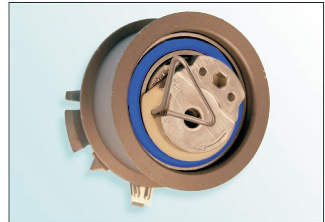
Рис. 2: 531 0565 30 (новая версия)
